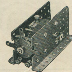
Moteur Electrique No. 1 (4 volts) Prix Frs. 112,00
