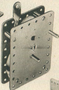
Moteur à Ressort N° 1A.
