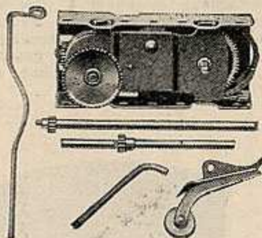
Moteur d'Avions à Ressort No. 2
