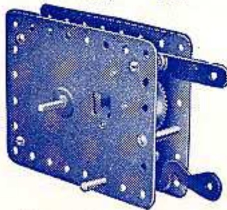
Moteur à Ressort No. 1
