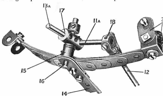
Fig. 6. Détail du pivot de direction côté gauche
