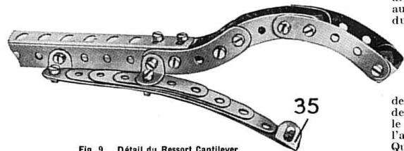
Fig. 9. Détail du Ressort Cantilever
