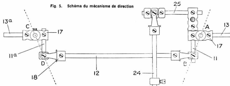
Fig. 5. Schéma du mécanisme de direction
