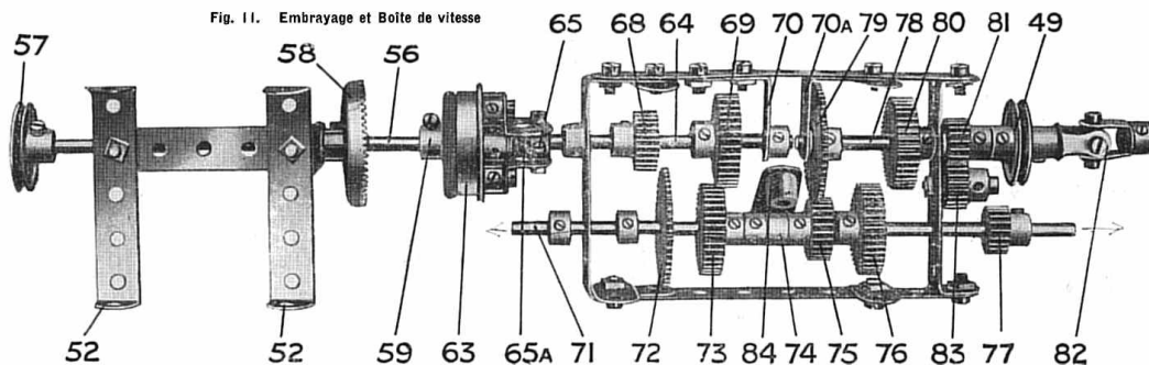
Fig. 11. Embrayage et Boîte de vitesse
