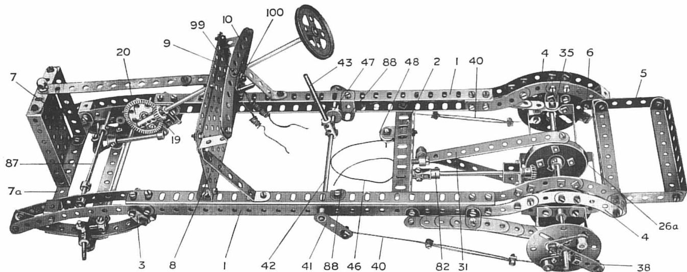
Fig. 2. Châssis montrant la suspension, le système de direction, les freins et le pont arrière dont le différentiel est enlevé
