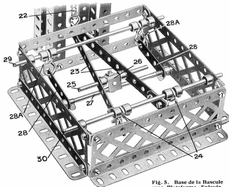
Fig. 5. Base de la Bascule avec Plateforme Enlevée.
