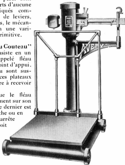
Fig. 2. Balance à Bascule Portable.
