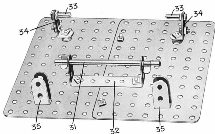
Fig. 4. Plateforme Vue de Dessous.
