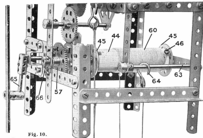
Fig. 10. Le mécanisme de remontage et la poulie du poids.
