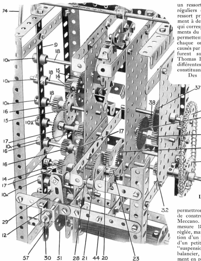
Fig. 9. Le train d'engrenages.
