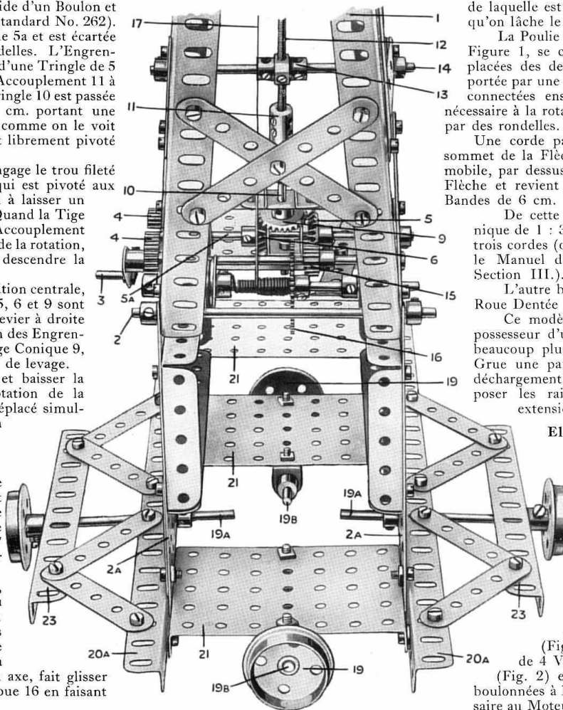
Fig. 4. Vue de devant de la Grue, montrant le mécanisme de hissage.
