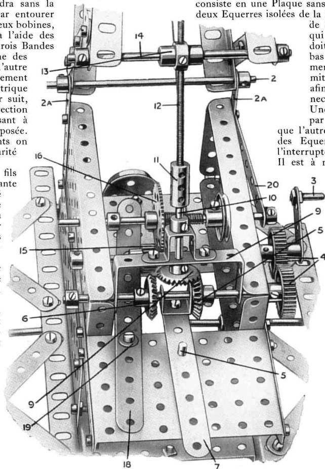
Fig. 5. La boîte de vitesse, vue d'arrière, montrant le mécanisme de levage avec le mécanisme de renversement, etc.
