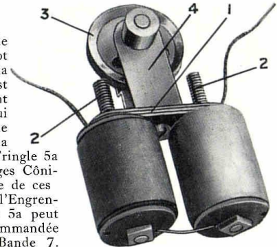
Fig. 3. L'électro-aimant Meccano.
