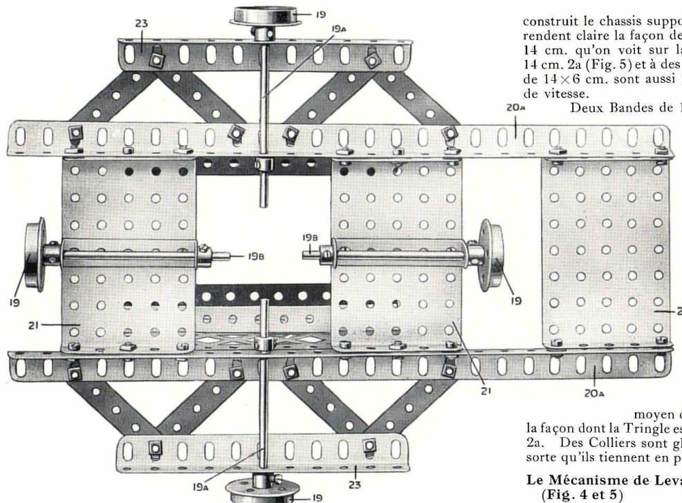
Fig. 2. Vue du dessous de la base du modèle, mettant en évidence la façon dont sont montés les axes des Roues. changement de vitesse. On voit mieux ces Bandes sur la Fig. 1. Les dispositifs de portants, soutenant les Tringles 19a (Fig. 2) sont constitués par des paires de Bandes de 6 cm. boulonnées aux Cornières 20a et aux Cornières 23 de 14 cm. Elles sont tenues en place par des Colliers et des Vis d'arrêt fixés à leurs extrémités intérieures contre les cotés intérieurs des Cornières 20a. Les extrémités extérieures des Tringles 19a portent les Roues à Boudin 19. Les Tringles 19b portant à leurs extrémités extérieures deux autres Roues à Boudin 19 passent à travers des Bandes Courbées de 60×12 mm. qui sont boulonnées au milieu des Plaques à Rebords 21 (voir la Fig. 2). Tout comme les Tringles 19a les Tringles 19b, sont maintenues en place à l'aide de Colliers glissés sur leurs bouts intérieurs et placés contre les Bandes Courbées. Ceci complète la construction de la plate forme de base, après quoi on
