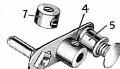
Fig. 9. Vue détaillée de la poignée du régulateur
