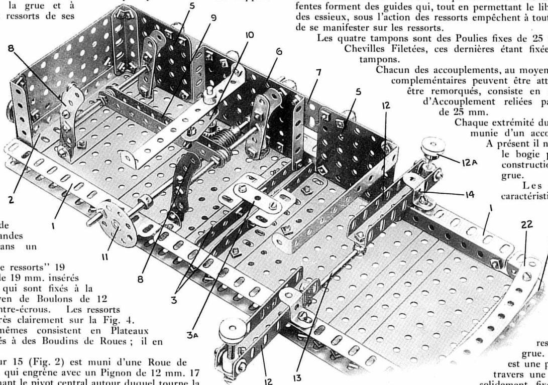
Fig. 3. Le châssis vu de dessous. Les parois latérales, et les roues locomotrices sont enlevées afin de faire voir les freins et les arcs-boutants coulissants.
