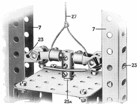
Fig. 5. Vue du toit de l'une des plates-formes-cabines entre les guides de la cage. Le câble de levage étant relâché, les cliquets du dispositif de sûreté s'engagent dans les trous des guides.
