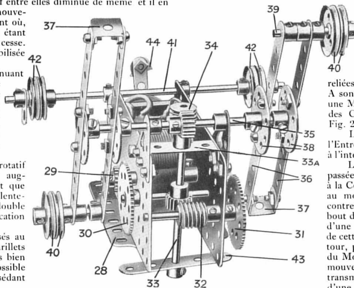
Fig. 8. Le mécanisme de levage.
