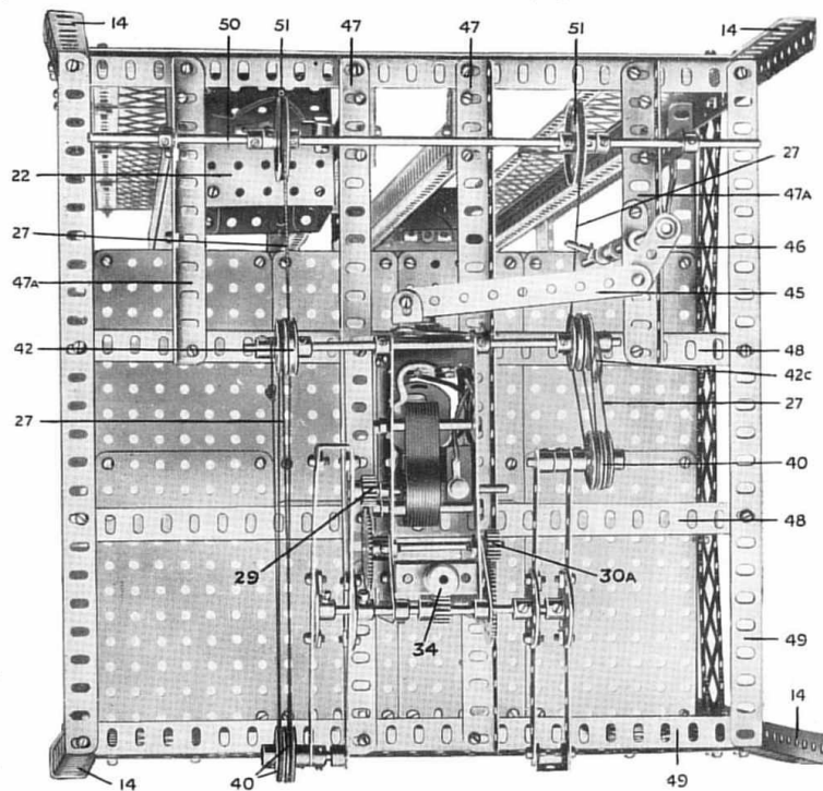
Fig' 7. Plan de l'étage supérieur de l'Entrepôt. Le toit est enlevé pour mettre à découvert le moteur et la machinerie.
