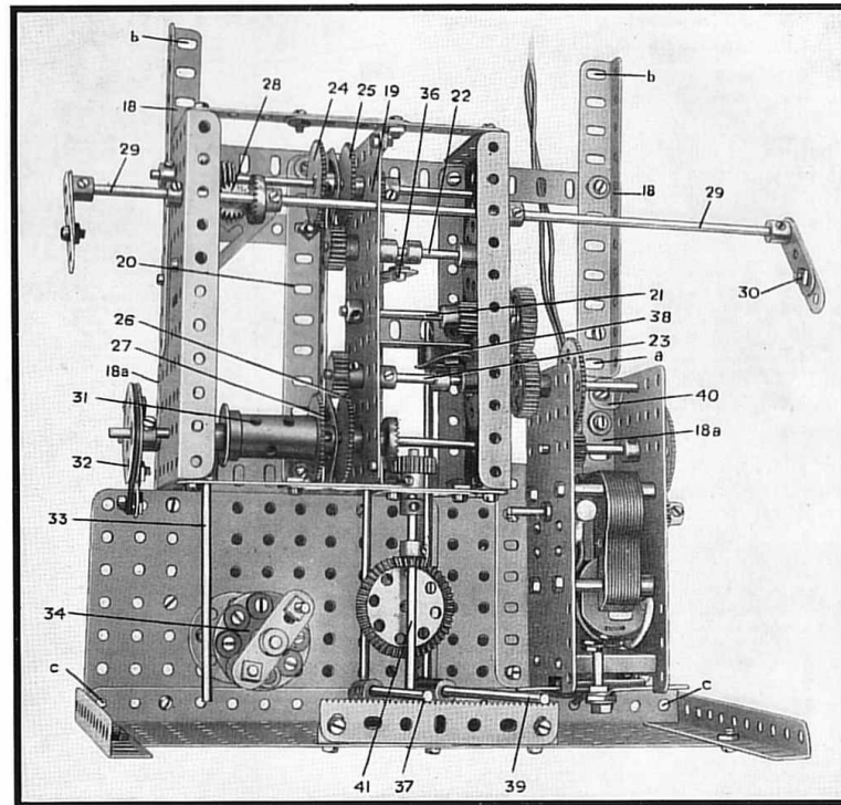
Fig. 5. La machine vue d'en haut.
