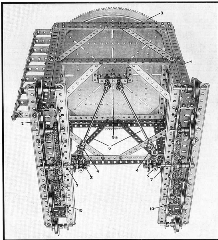
Fig. 3. Le portique du modèle vu d'en dessous.
