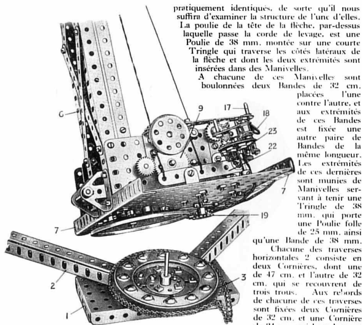
Fig. 3. Vue de la plate-forme pivotante et de la machinerie, montrant le Roulement à Billes.
