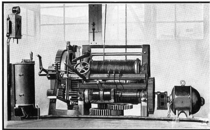
Fig 4. La machinerie d'une véritable grue derrick.
