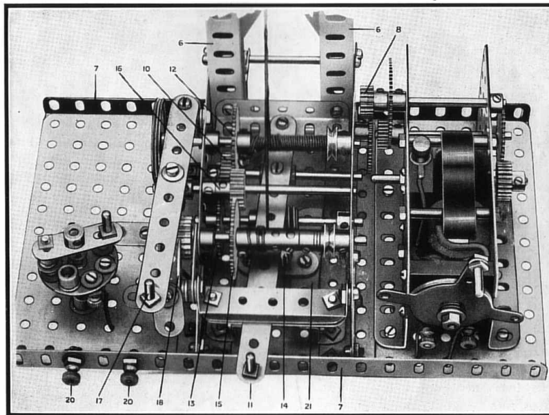
Fig 5. Vue de dessus de la machinerie du modèle faisant voir les engrenages, le Moteur Electrique, les leviers de commande, les freins, le régulateur, etc.
