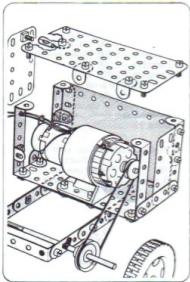
1. entraînement par poulie
