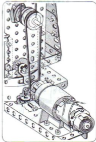
3. entraînement vertical avec renvoi de poulies
