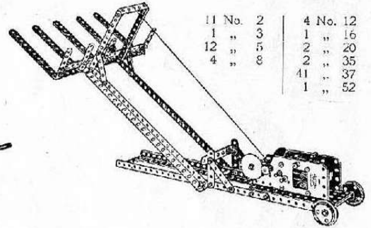
Hay Stacker Faneuse
