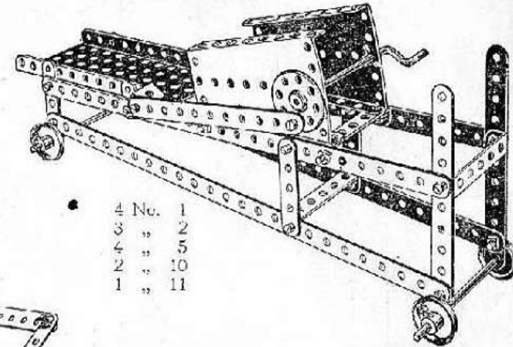
Maize Sheller Décortiqueuse
