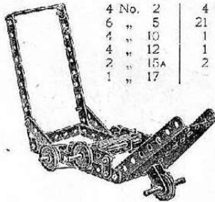
Music Stand Pupitre à Musique
