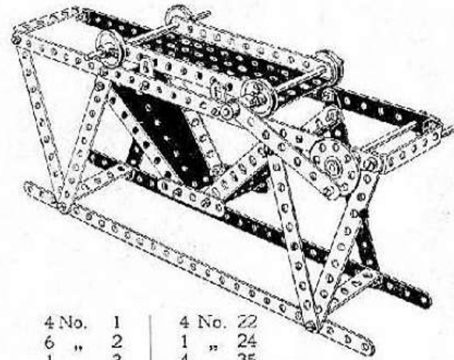
Sifter Tamiseur
